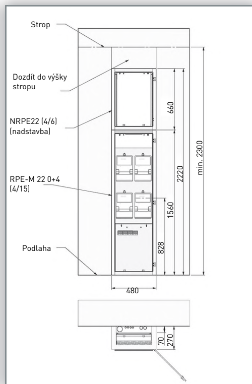
Sestava rozvodnice RPE-M + NRPE s požární odolností EW 30 Možné použití pro snížené stropy s minimální výškou 2300 mm
