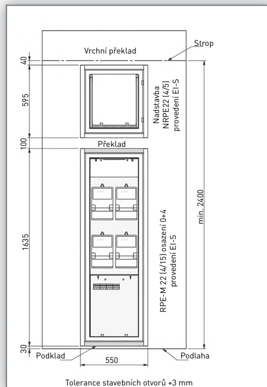
Sestava rozvodnice RPE-M + NRPE s požární odolností EI-S Možné použití pro snížené stropy s minimální výškou 2400 mm
