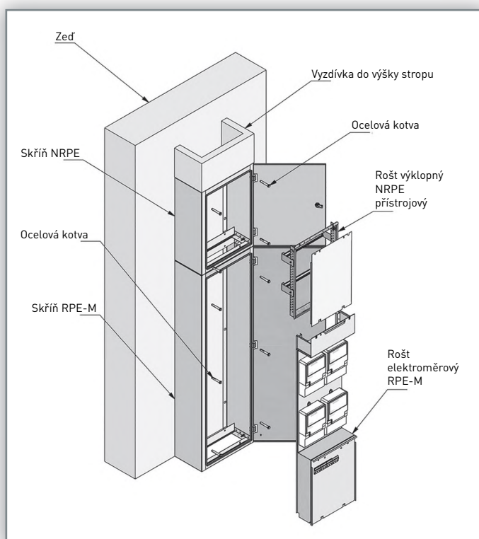
Sestava rozvodnice RPE-M + NRPE s požární odolností EW 30 Možné použití pro snížené stropy s minimální výškou 2300 mm
