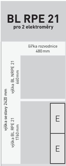
Tabulka elektroměrových rozvodnic BL-RPE s požární odolností EW 30
