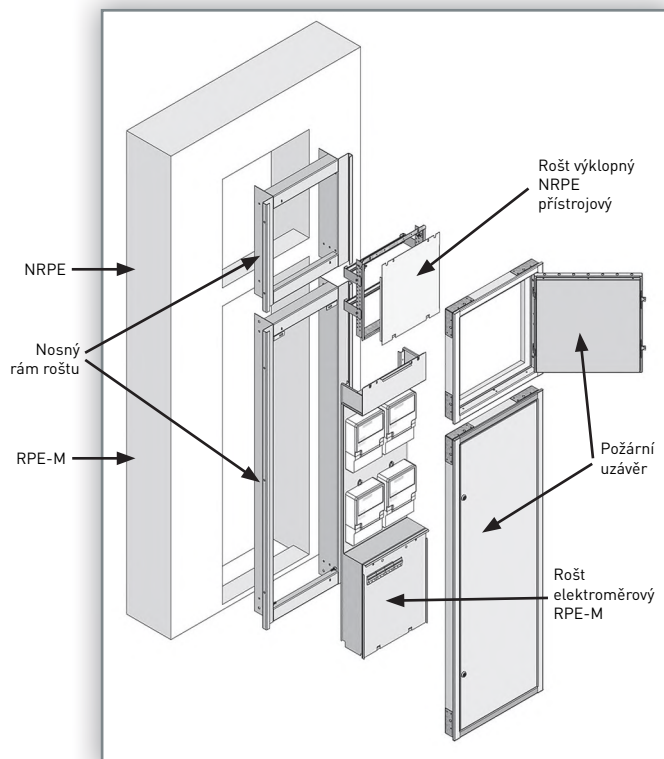
Sestava rozvodnice RPE-M + NRPE s požární odolností EI-S Možné použití pro snížené stropy s minimální výškou 2400 mm
